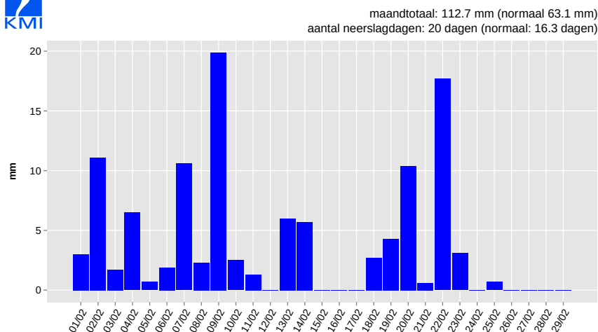
Dagelijkse neerslaghoeveelheid, Ukkel, februari 2016
