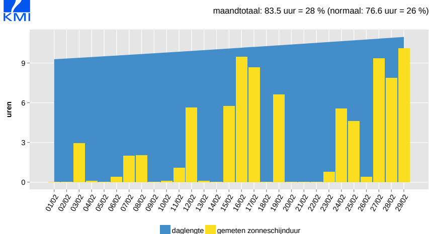
Dagelijkse zonnenschijnduur, Ukkel, februari 2016
