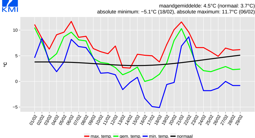
Dagtemperatuur, Ukkel, februari 2016
