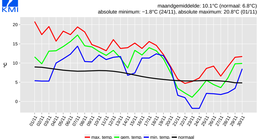
Dagtemperatuur, Ukkel, november 2015
