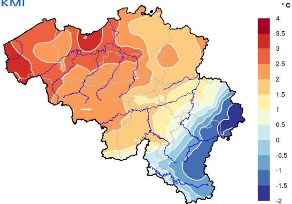
Dagelijkse minimumtemperatuur gemiddelde januari 2016
