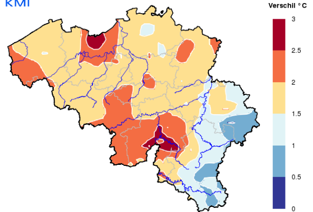
Afwijking van de normaalwaarde van de dagelijkse minimumtemperatuur gemiddelde januari 2016 in vergelijking met de maandelijkse normaalwaarde 1981-2010
