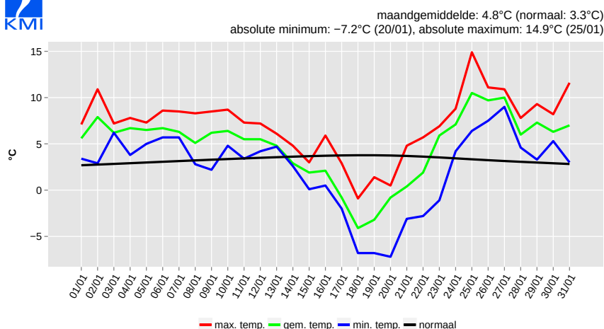
Dagtemperatuur, Ukkel, januari 2016
