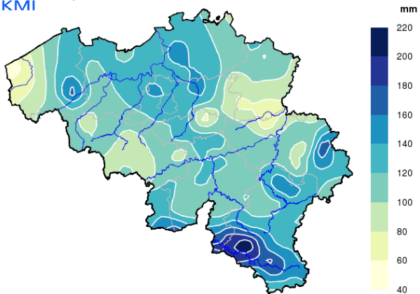
Neerslaghoeveelheid totaal januari 2016
