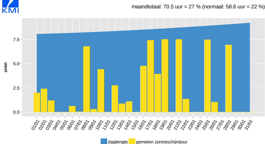
Dagelijkse zonschijnduur, Ukkel, januari 2016
