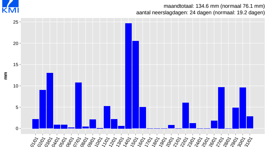
Dagelijkse neerslaghoeveelheid, Ukkel, januari 2016
