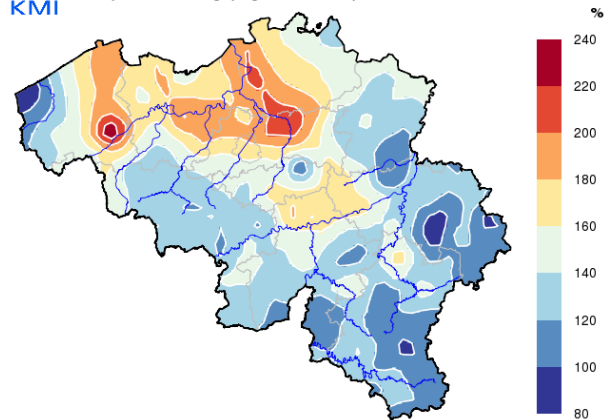
Verhouding tot de normaalwaarde neerslaghoeveelheid totaal januari 2016 in vergelijking met de maandelijkse normaalwaarde 1981-2010
