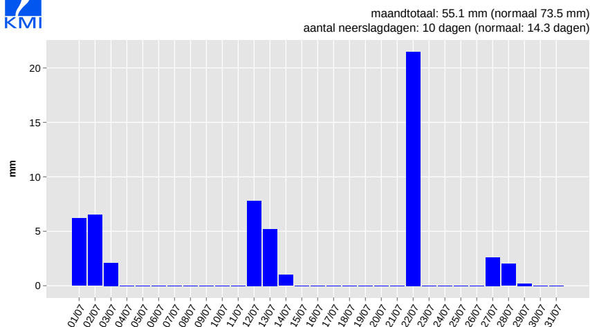
Dagelijkse neerslaghoeveelheid, Ukkel, juli 2016
