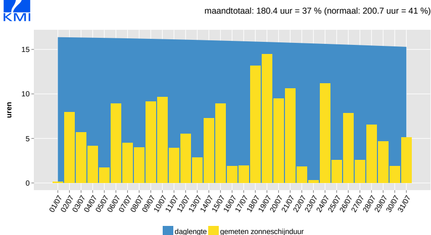
Dagelijkse zonschijnduur, Ukkel, juli 2016
