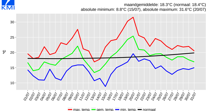
Dagtemperatuur, Ukkel, juli 2016
