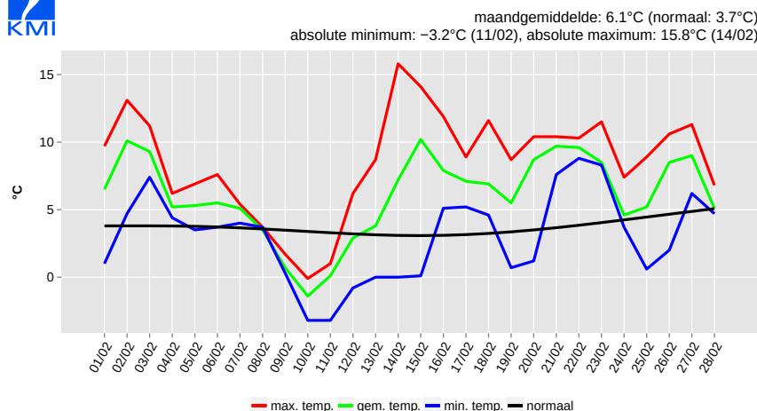
Dagtemperatuur, Ukkel, februari 2017
