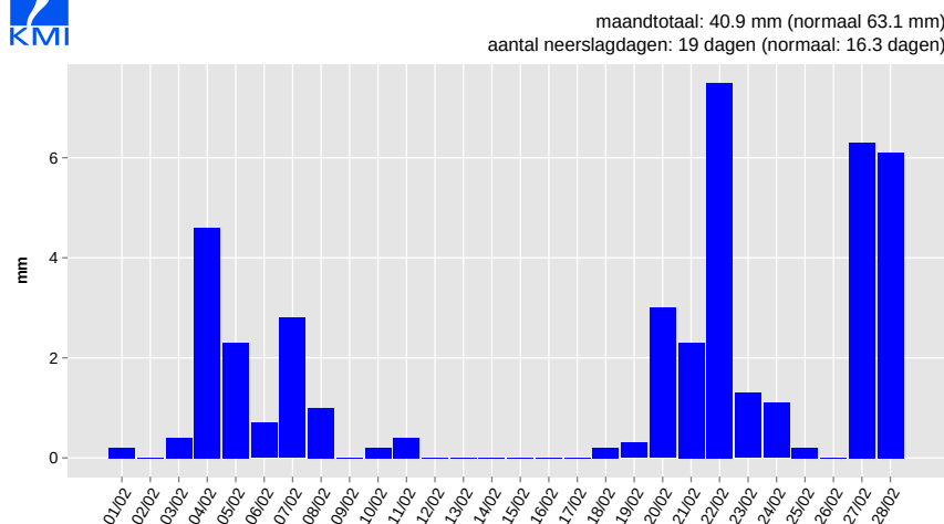
Dagelijkse neerslaghoeveelheid, Ukkel, februari 2017
