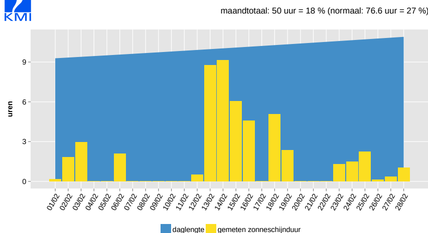
Dagelijkse zonschijnduur, Ukkel, februari 2017
