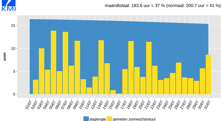
Dagelijkse zonschijnduur, Ukkel, juli 2017
