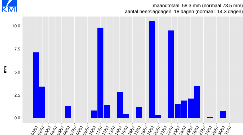
Dagelijkse neerslaghoeveelheid, Ukkel, juli 2017
