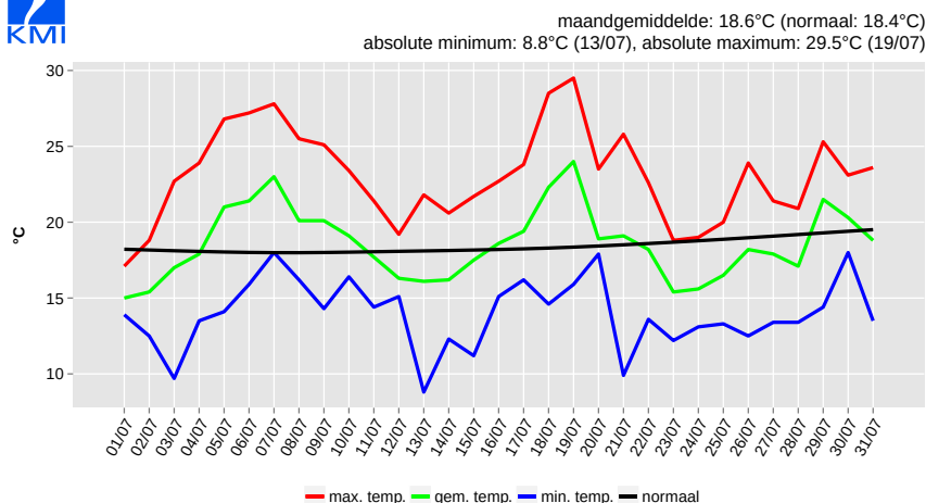
Dagtemperatuur, Ukkel, juli 2017
