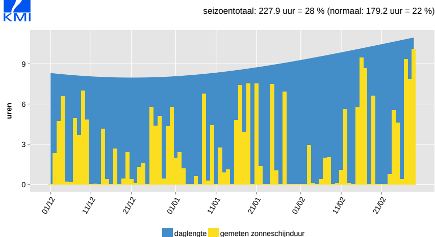
Dagelijkse zonschijnduur, Ukkel, winter 2016
