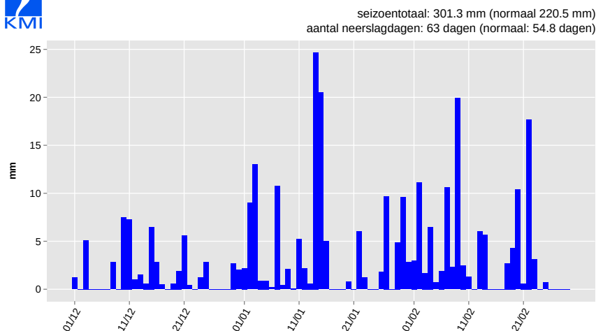
Dagelijkse neerslaghoeveelheid, Ukkel, winter 2016
