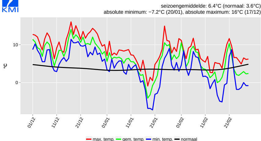
Dagtemperatuur, Ukkel, winter 2016
