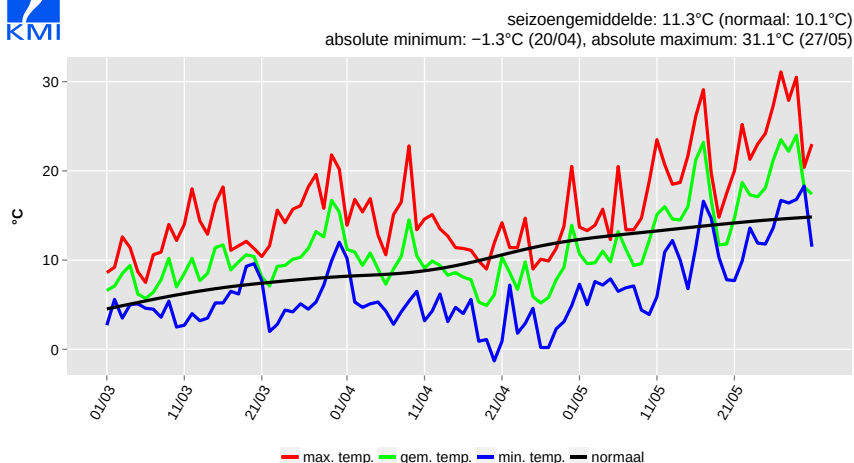
Dagtemperatuur, Ukkel, lente 2017
