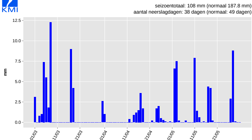
Dagelijkse neerslaghoeveelheid, Ukkel, lente 2017
