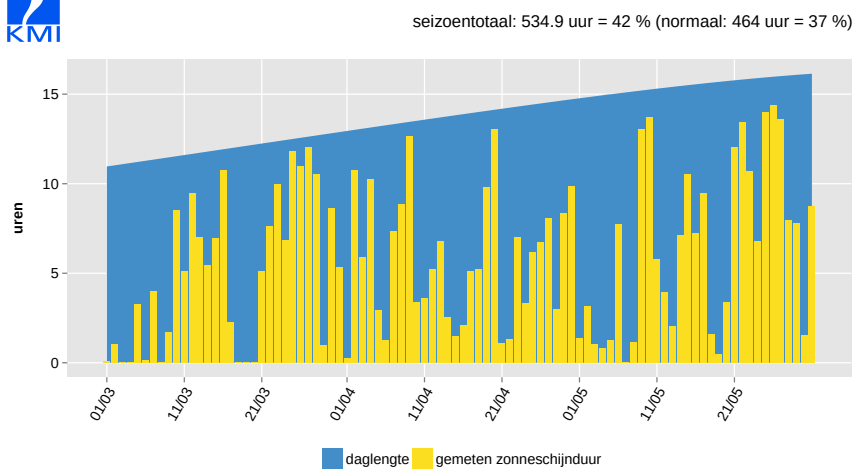
Dagelijkse zonschijnduur, Ukkel, lente 2017
