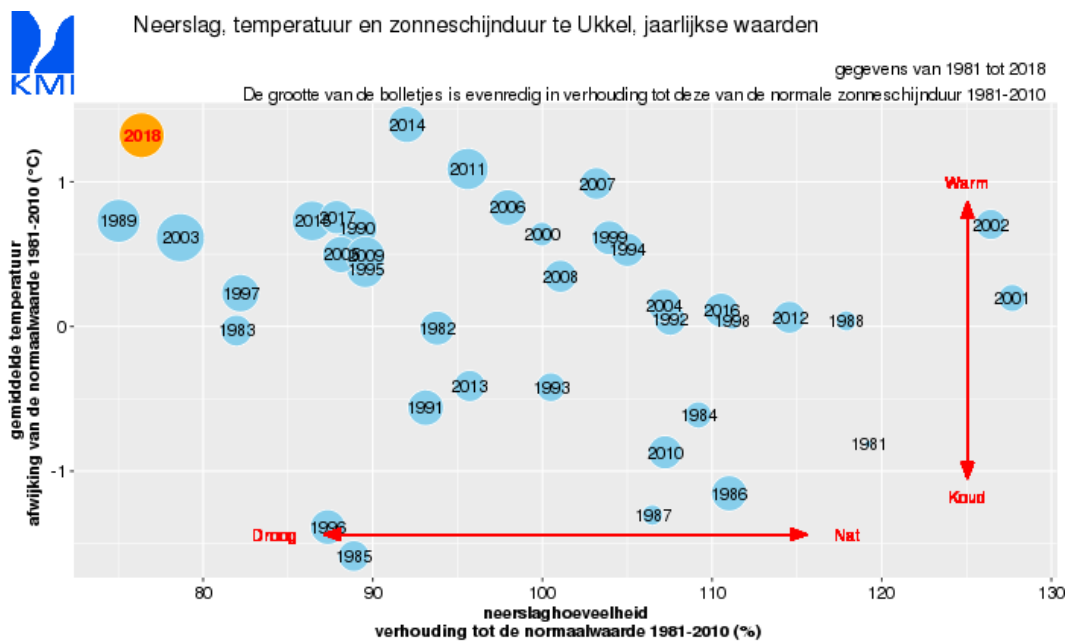
Figuur 1: Positie van het jaar 2018 voor de gemiddelde temperatuur, de neerslaghoeveelheid en de zonneschijnduur (vanaf 1981).
